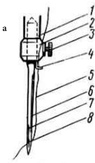
Расми 36 Навъҳои сӯзани мошини дарздӯзӣ
