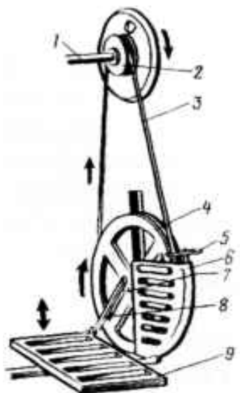
Расми 34 ҳаракатовари поякии мошинаи дарздӯзӣ 1- чархи асосӣ 2-шкиви чархи гардона 3-тасма 4-чархи ҳаракатдиҳанда 5-тасмагардон 6-сипарча 7-кривошип (танзимаи ҳаракат 8- шатун 9-педал
